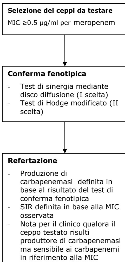
Figura 2 - Algoritmo per l'identificazione fenotipica e la refertazione degli enterobatteri produttori di carbapenemasi
